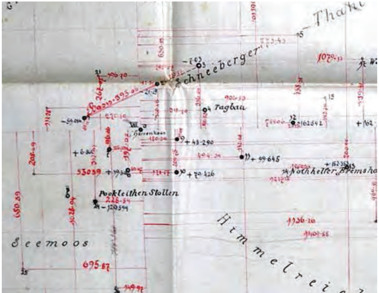
Abbildung 17: Ausschnitt aus der Abschrift eines Punktauftrags „Triangulierungsnetz von Schneeberg“, mit Markierung des Koordinatennullpunkts (= TP 8) und der Basislinie im Tal nahe der Bergschmiede. Originalmaßstab 1:10.000 (hier vergrößerter Ausschnitt), rechts unten (im Bild nicht sichtbar) signiert bzw. datiert „Zieglheim“ sowie „cop[iert] Jos. Billek 23.3.1891 Copirt 5. Jänner 1893 Hantinger“ (letzter Name unklar). Schneebergarchiv des Südtiroler Bergbaumuseums, Inv.-Nr. 382. 18
