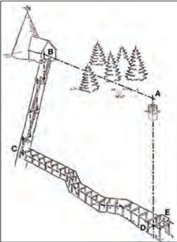
Abbildung 6: Prinzip des Fällens von Lochsteinen in die Grube: Die Koordinaten eines Lochsteins, der überragt eine Grubenfeldgrenze markiert, werden über Polygonzüge, ggf. mit Schachtlotungen, in die Grube übertragen und an der Stelle in der Strecke, die lotrecht unter dem Lochstein liegt, die Erbstufe geschlagen. Quelle: Herbert Denner, Lochsteine, Clausthal-Zellerfeld 1984, Abb. 4a auf S. 10
