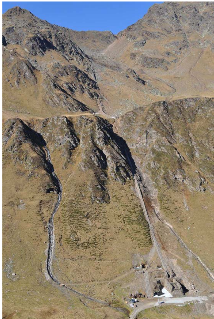
Abb. 1: Teilbereich der Erzüberbrückungsanlage im Ridnaun. Rechter unterer Eckbereich der Untere Lazzacher Erzkasten. Darüber der untere Teilbereich des Lazzacher Bremsbergs (CONTEXT OG).
